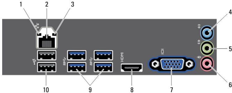
圖 2. 背面板視圖
